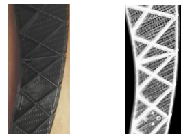
Contrôle de défauts sur matériau composite à renforts tissés
