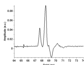
Mesure d'épaisseur d'un carbone epoxy avec coating multicouche
