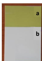
Mesure d'épaisseur d'un carbone epoxy avec coating multicouche
